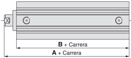
Doble efecto, Vástago simple/ Carrera larga
