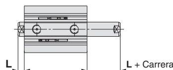
Rosca hembra terminación vástago
