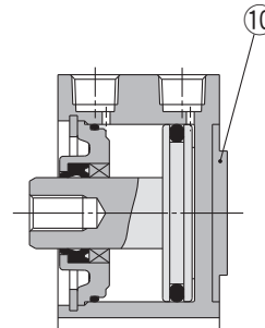
Con muñón posterior de centrado
