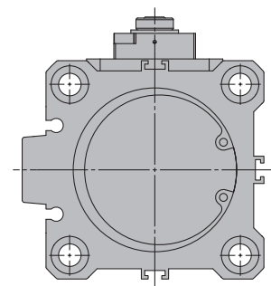
Forma de la camisa del cilindro Ø 80 mín.
