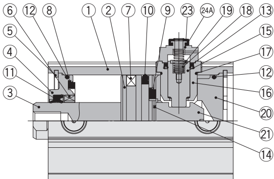
Bloqueo trasero
