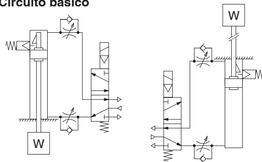
Con bloqueo en extremo posterior
