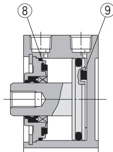
Con tope elástico
