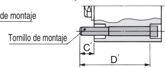
Montaje en el lado del vástago
