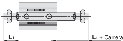
Rosca macho en extremo del vástago
