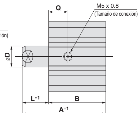
Muelle extendido
