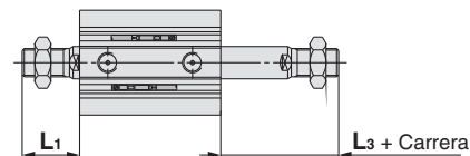
Rosca macho en extremo del vástago
