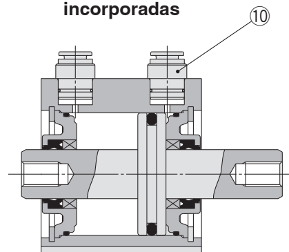
Conexiones instantáneas incorporadas
